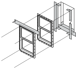
凸缘窗 选项2－低度暴露
