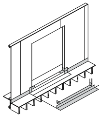
有装饰的外门
