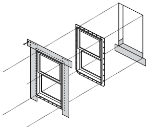
凸缘窗 选项1－低度暴露
