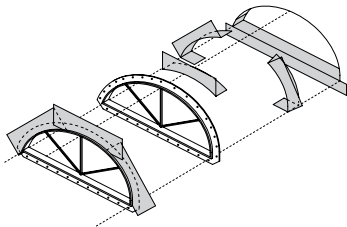
半圆窗 选项2－重度暴露
