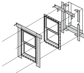
凸缘窗 选项3－低度暴露
