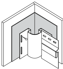
墙到墙 内角
