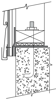
基槛板 选项1
