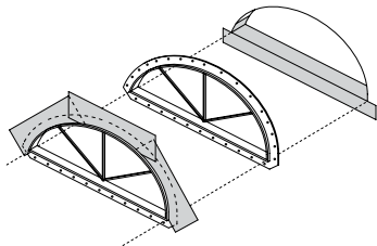
半圆窗 选项1－低到中度暴露
